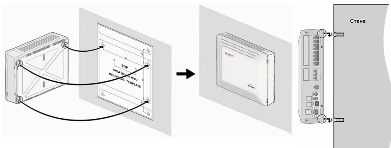
Рис. 2.6 Настенный монтаж базового блока
