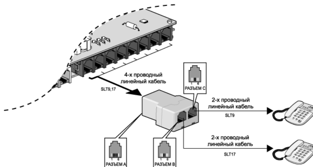
Рис. 2.14 Терминальный переходник
