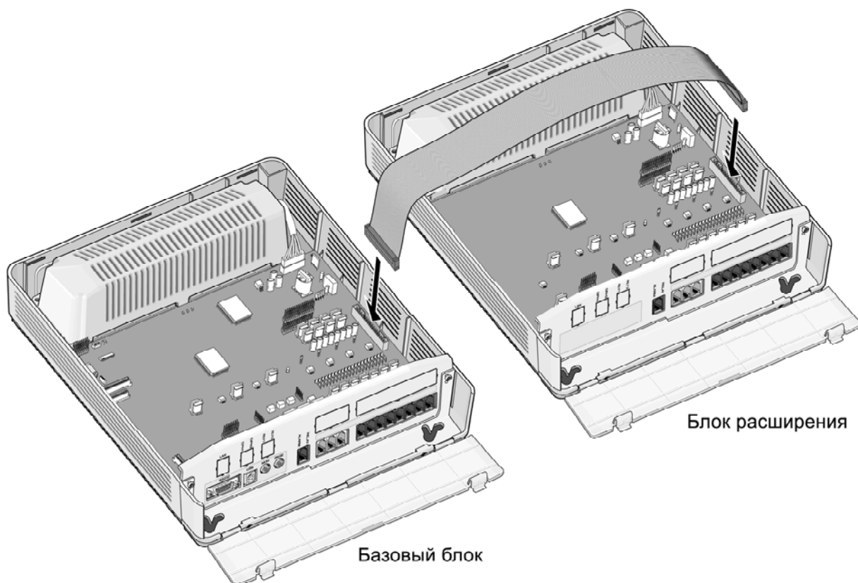
Рис. 2.8 Подключение блока расширения к базовому блоку
