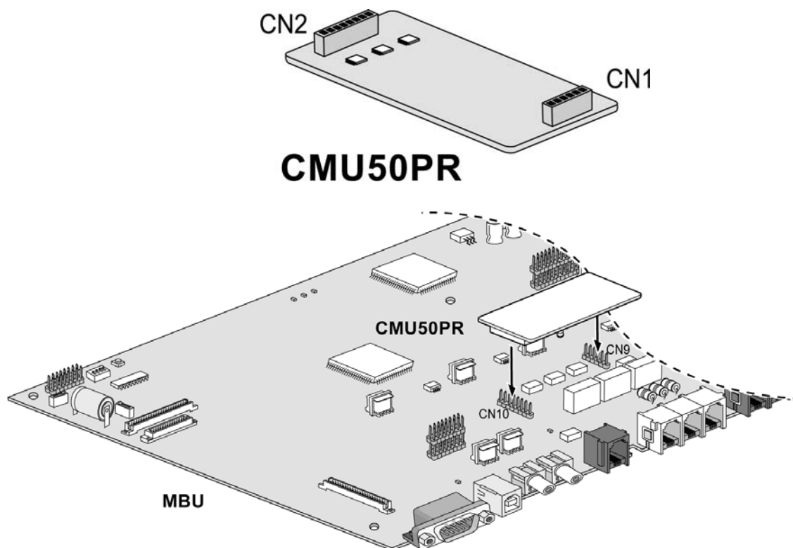
Рис. 2.20 Модуль определения импульсов тарификации CMU50PR
