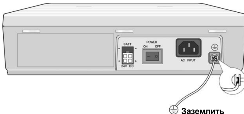
Рис. 2.3 Заземление корпуса
