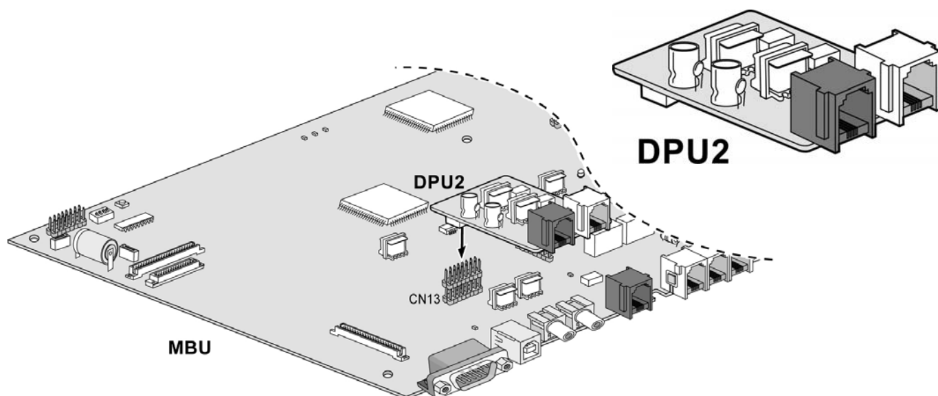
Рис. 2.19 Модуль для подключения домофона DPU2
