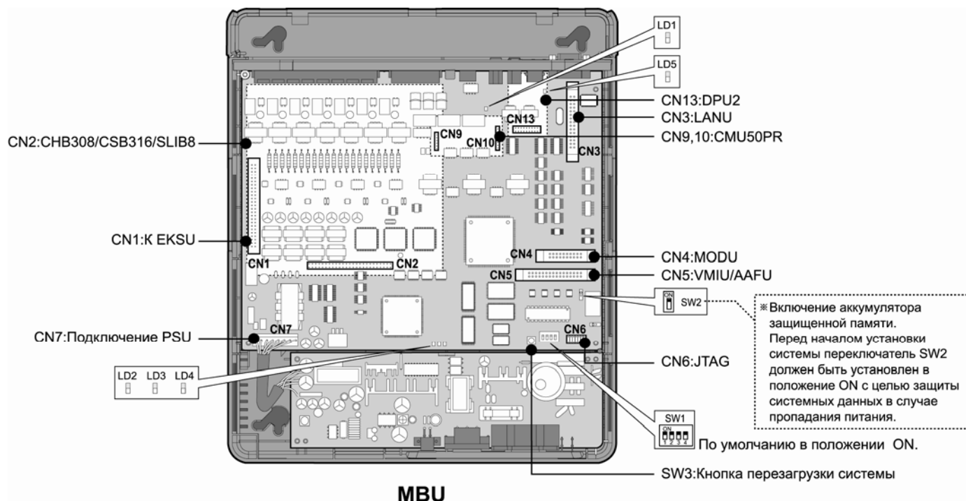
Рис. 2.10 Материнская плата базового блока (MBU)
